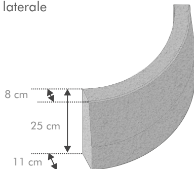
vista laterale
